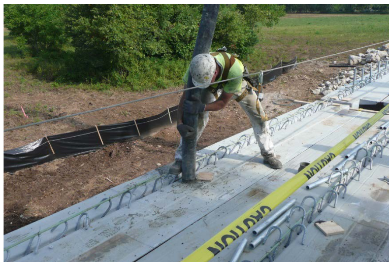
Figure 3-13 B0478 In-Situ Concrete Pour
